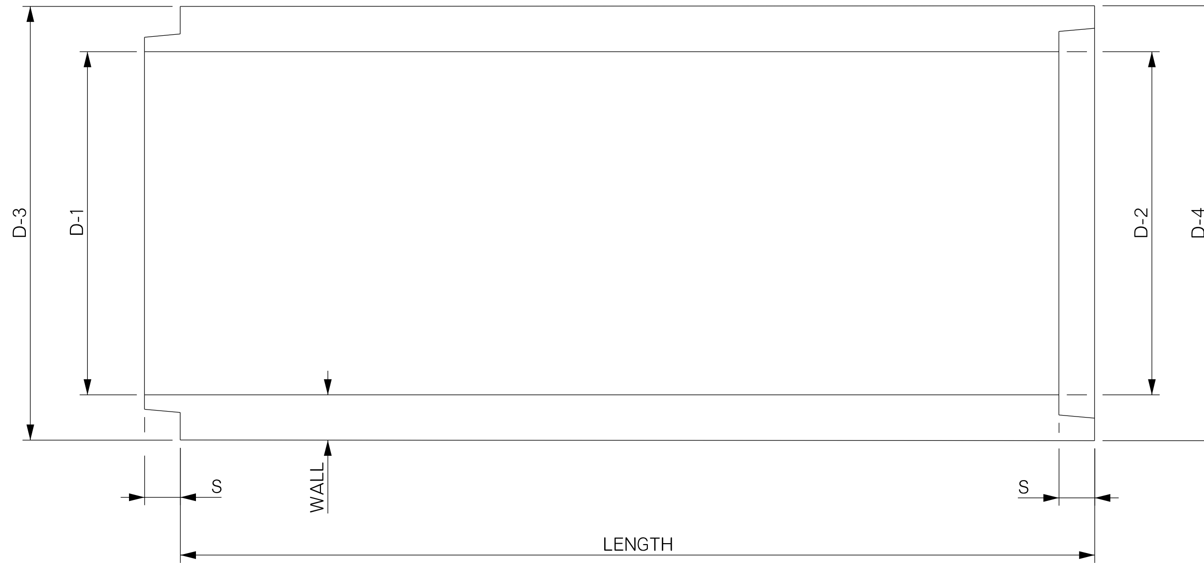
ELEVATION
